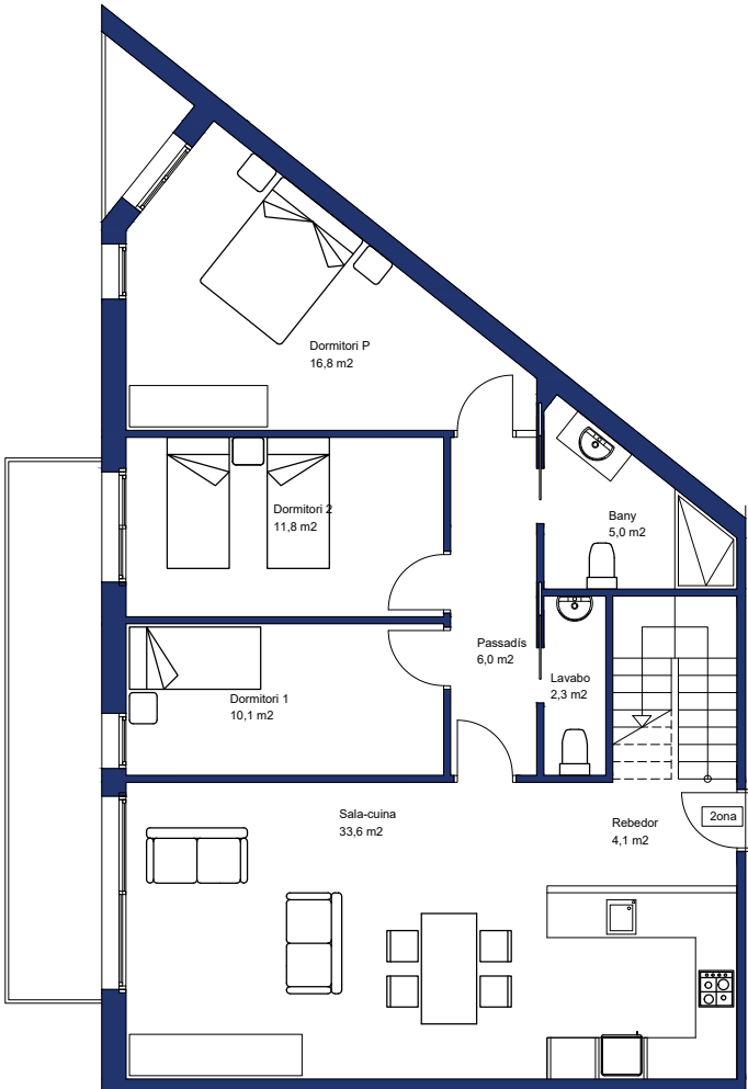
PLANTA SEGONA
