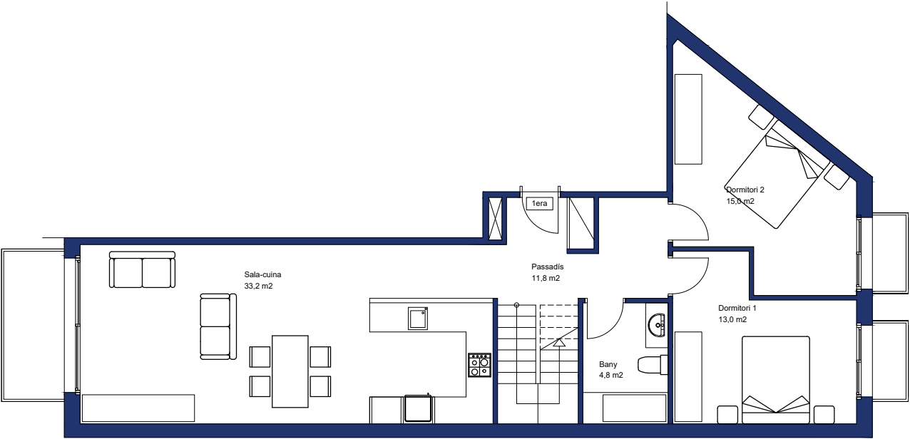
PLANTA SEGONA
