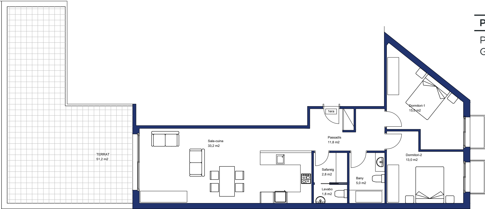
PLANTA PRIMERA
